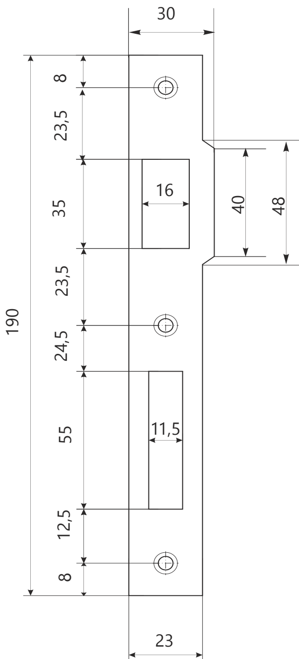
Ответная планка
