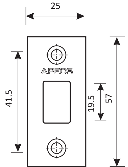
Ответная планка
