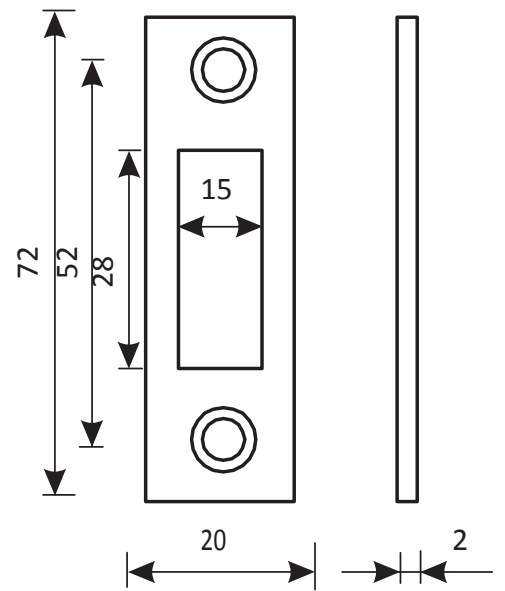
Ответная планка
