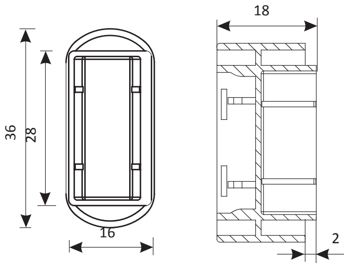
Вкладыш под ответную планку
